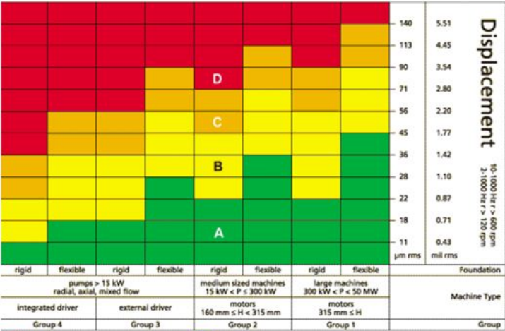
ISO-10816-3 - DISPLACEMENT
